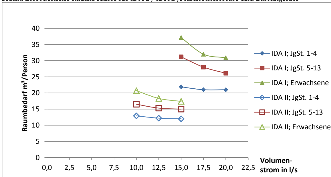
Graphik: Erforderliche Raumbedarfe für IDA 1 / IDA 2 je nach Altersstufe und Lüftungsrate
